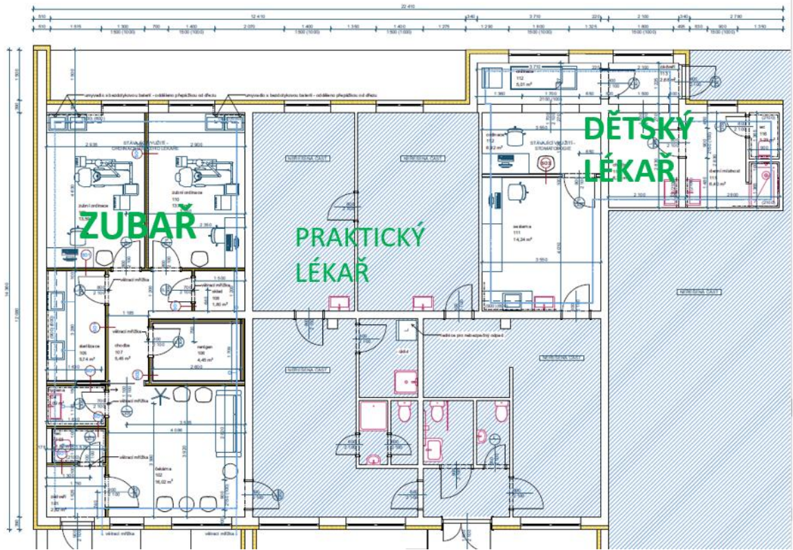
PŮDORYS 1.NADZEMNÍ PODLAŽÍ - nový stav
