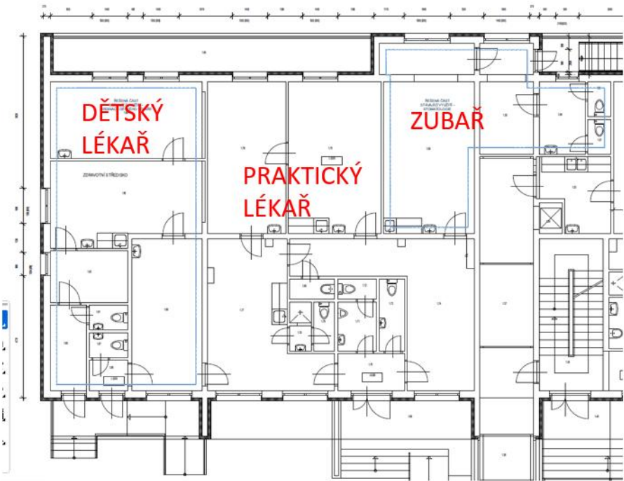
PŮDORYS 1.NADZEMNÍ PODLAŽÍ - stávající stav
